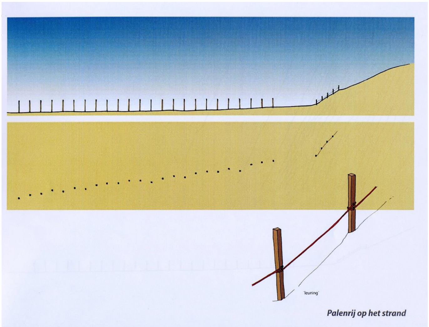
Ontwerp palenrij om het gebied op strand en in de reep te markeren
